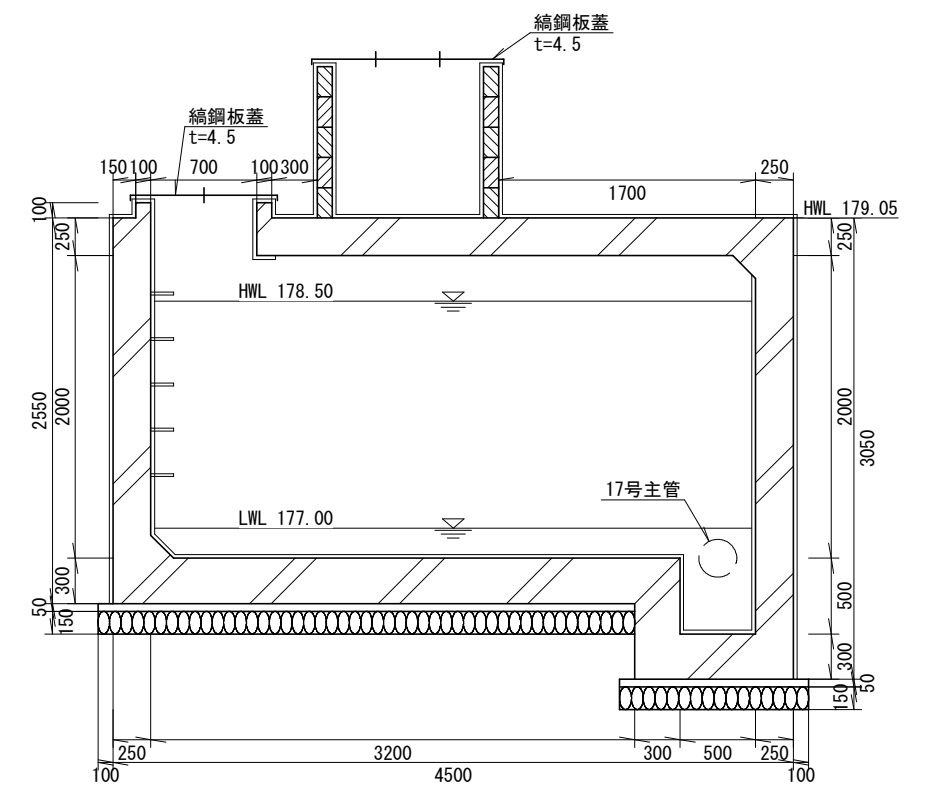
A—A 断面图
