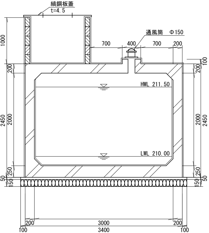
B-B断面図
