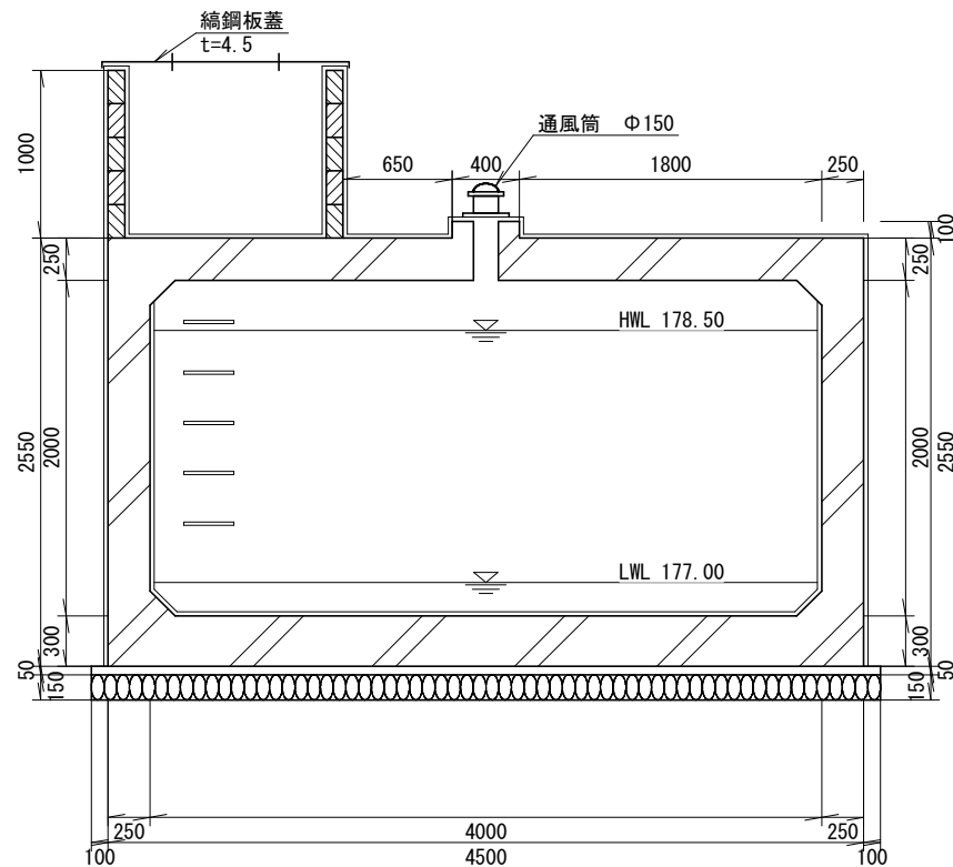
B—B 断面图
