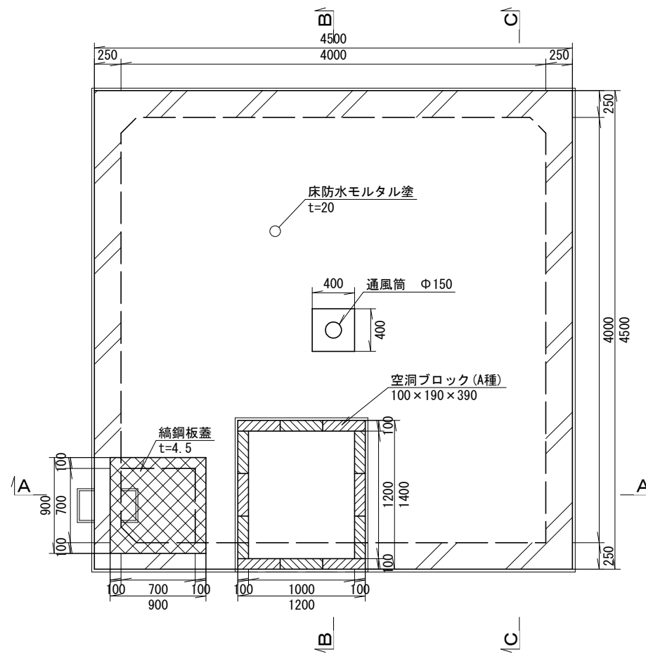
床版平面図
