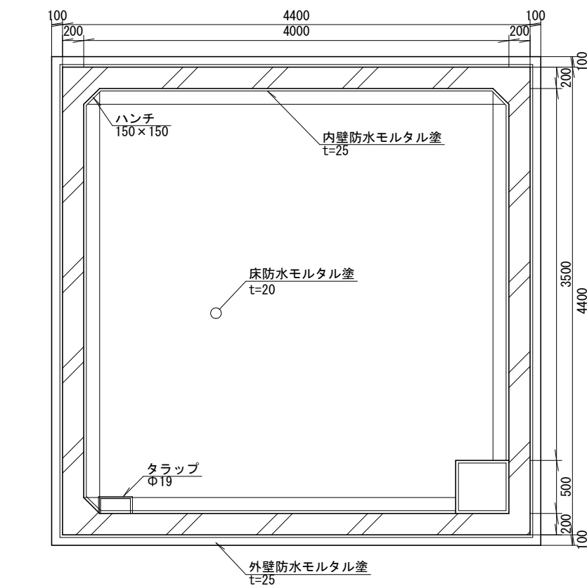
底板平面図
