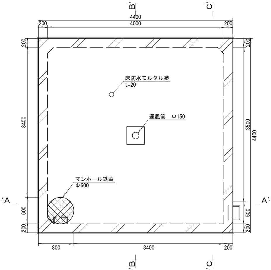
床版平面図
