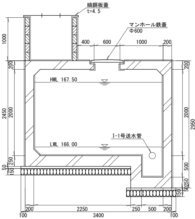
A-A断面図
