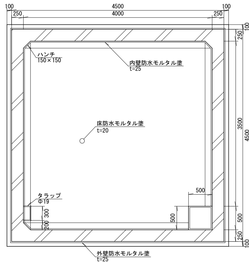
底版平面图
