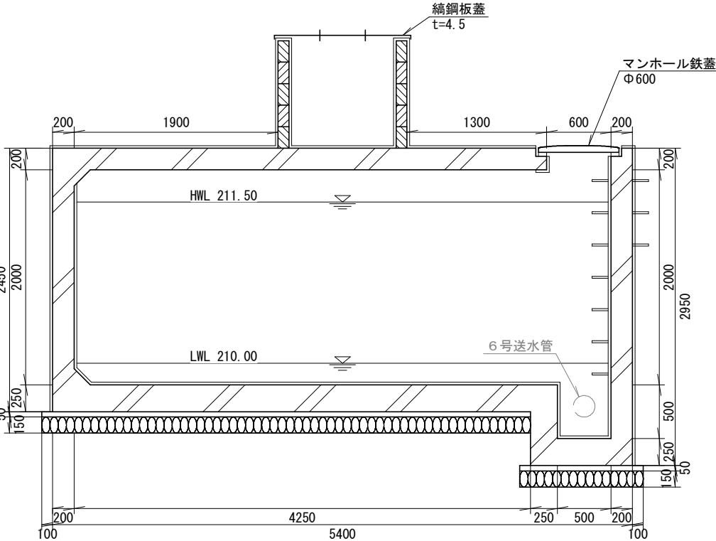
A-A断面図
